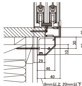
ふかし枠50タイプ
