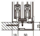
ふかし枠50タイプ
