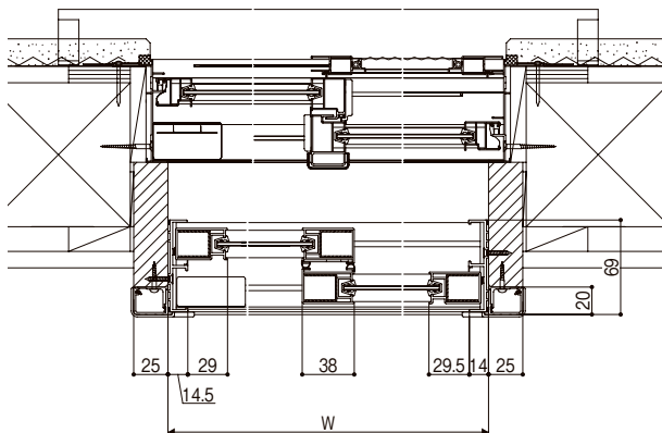
横断面図
