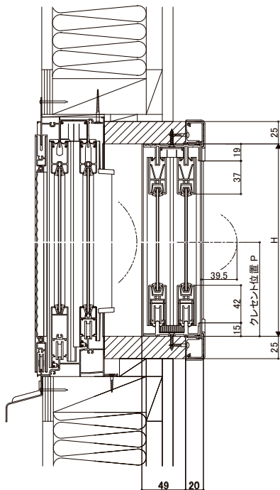
ふかし枠20タイプ
