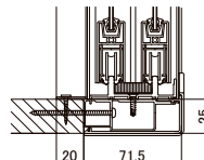
ふかし枠70タイプ
